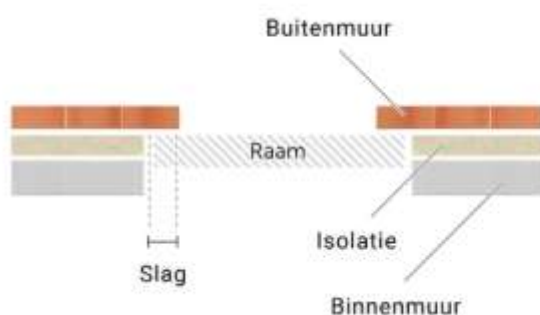
Spouwmuur met slag (veel voorkomend)
